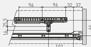
Prowadnica rolkowa / Euro roller slide / Роликовая направляющая
